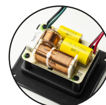
Diskrete Frequenzweiche
